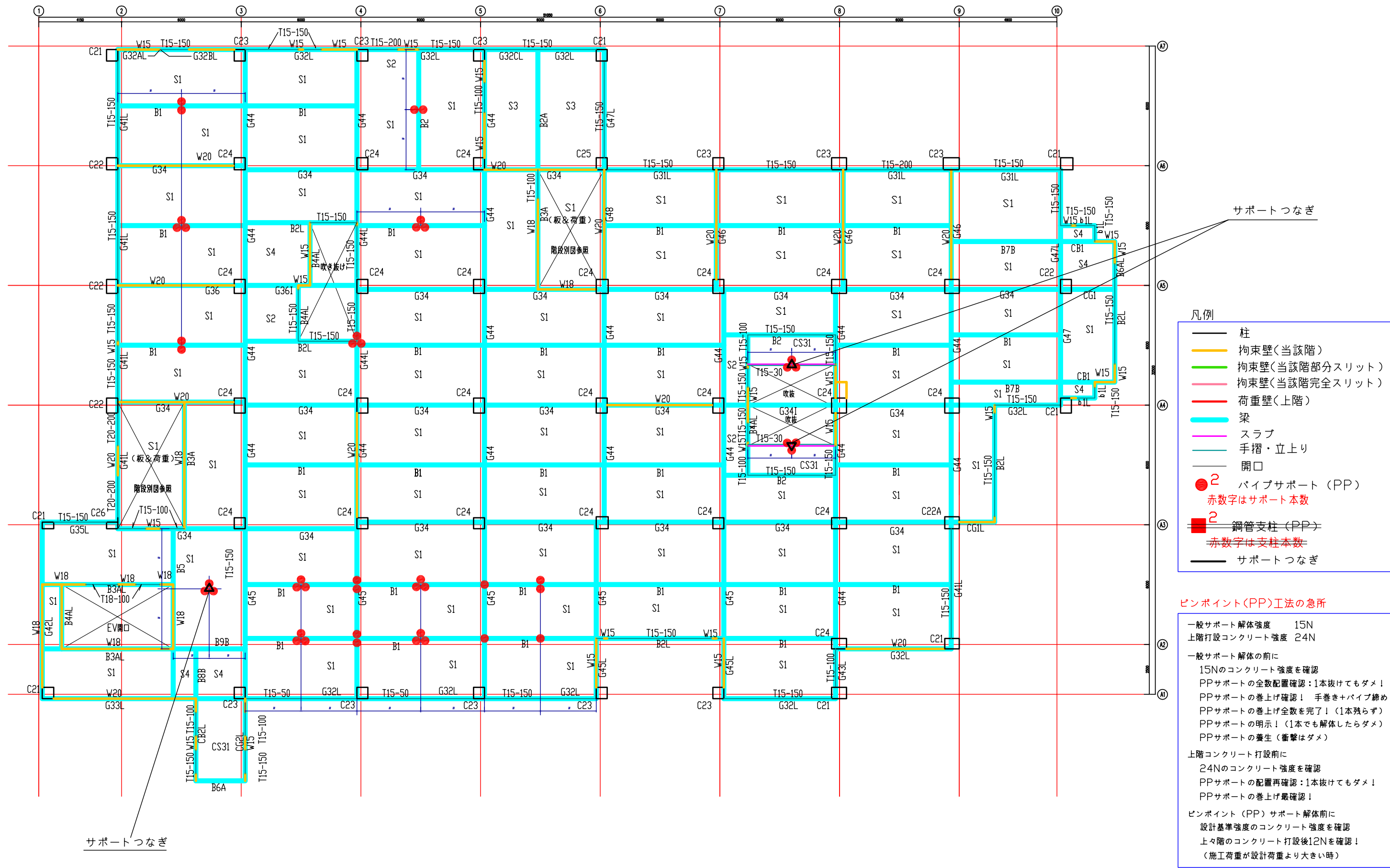
型枠支保工早期解体計画図 (ピンポイント工法: FEM解析による)
