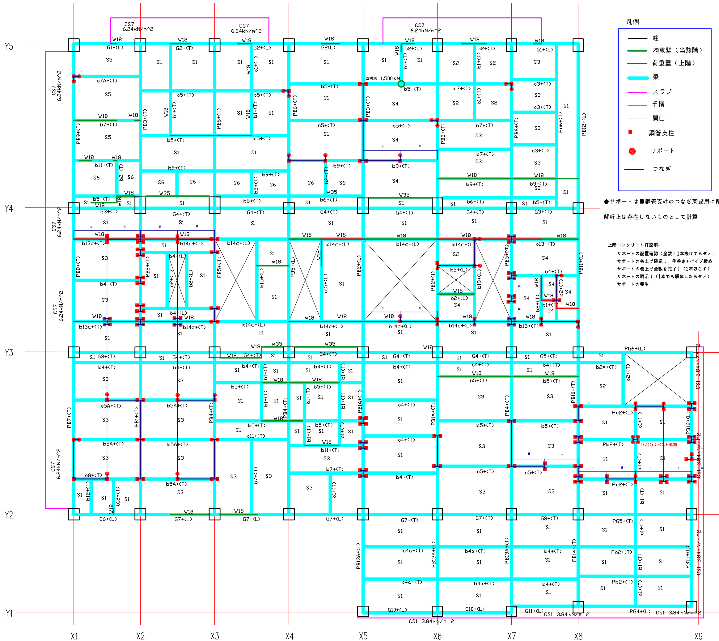
消防局庁舎 型枠支保工解体計画 (1階柱壁2階梁スラブ) パーマネントサポート配置図 [FEM解析による]
